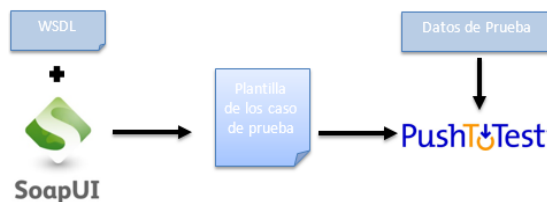
Figura 6. Proceso de inyección de datos Fuente: Elaboración propia.
