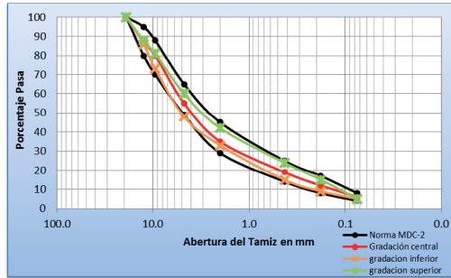
Figura 3. Franjas Granulométricas de las tres mezclas, Central, Inferior y Superior
